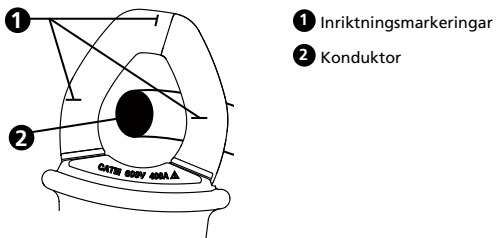
Figur 2: Inriktningssmarkeringar
