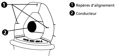
Fig. 2 : Repères d'alignement
